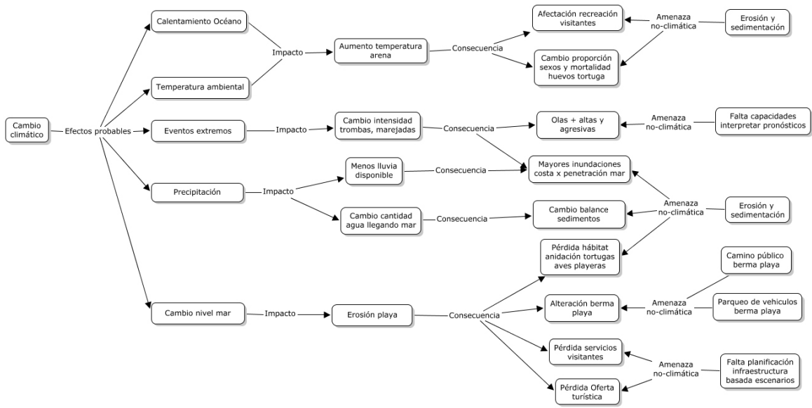
Figura 3. Cadena de impacto climático en el sistema de playas del Refugio Nacional de Vida Silvestre Playa Hermosa-Punta Mala
